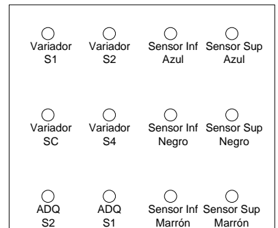
Ficha Macho Vista Frontal
